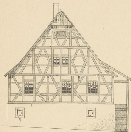
Abb. 1. Vorderansicht des Wirtschaftshauses.
