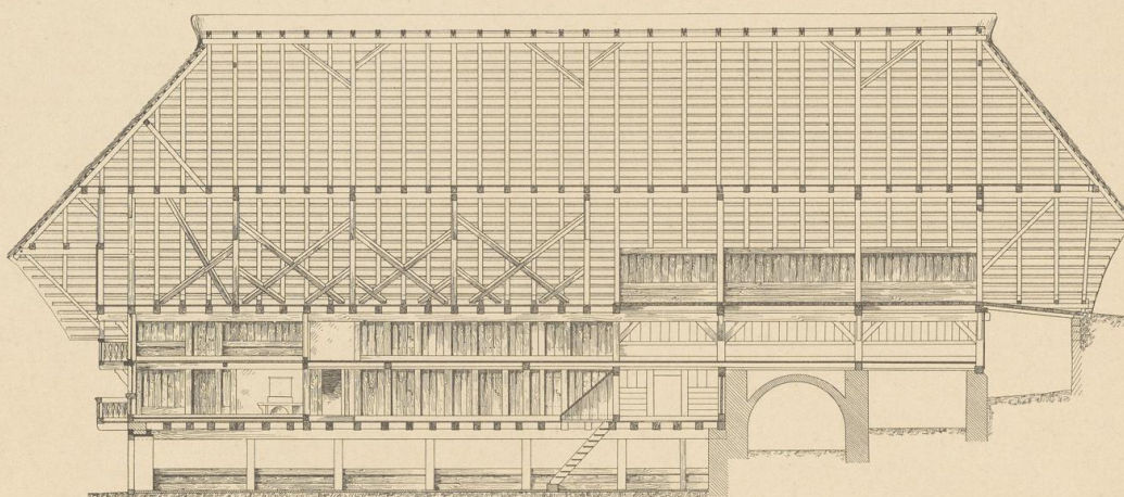
Abb. 2. Längenschnitt A B.
