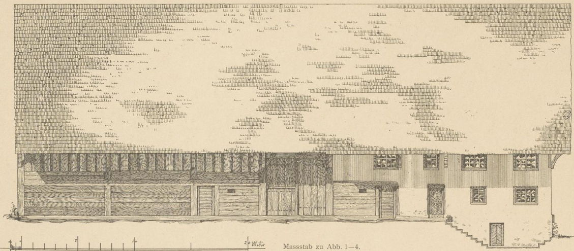
Abb. 1. Vordere Längsansicht.
