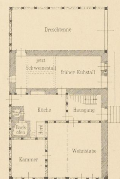
Abb. 6. Grundriss vom Erdgeschoss.
