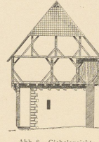
Abb. 8. Giebelansicht. Ursprünglicher Zustand.
