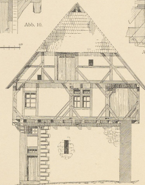
Abb. 4. Giebelansicht.
