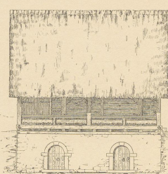
Abb. 8. Ansicht gegen das Thal. Speicherbau.
