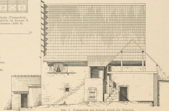
Abb. 5. Südansicht mit Schnitt durch die Scheune.
