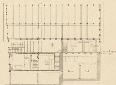
Abb. 4. Herbolzheim. Längenschnitt.
