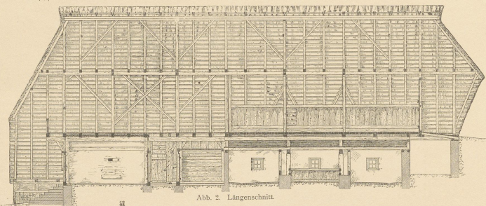
Abb. 2. Längenschnitt.
