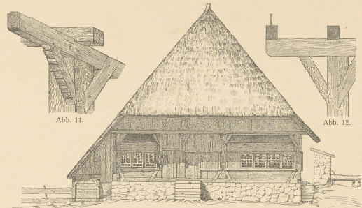
Abb. 3. Ansicht gegen das Thal.
