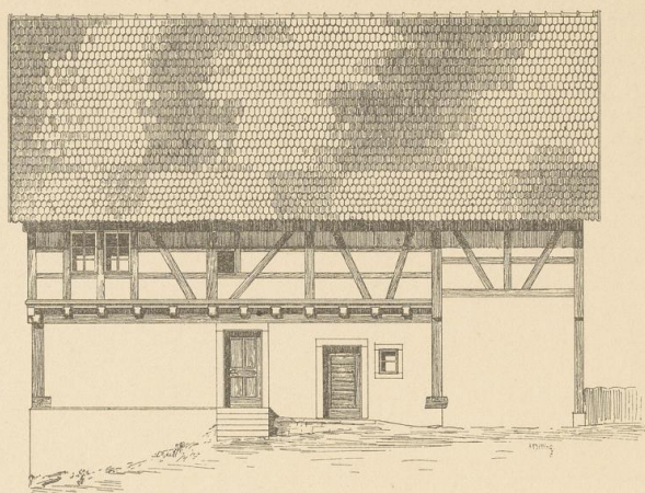
Abb. 2. Seitenansicht.
