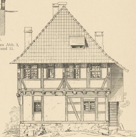
Abb. 6. Kippenheim Nr. 227. Hintergiebel.
