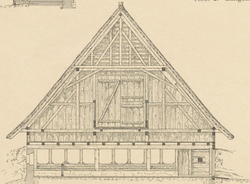
Abb. 7. Schnitt B-C.
