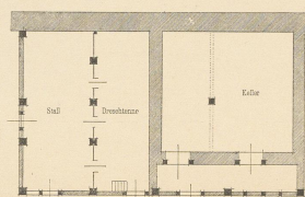
Abb. 7. Grundriss des Untergeschosses.
