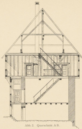
Abb. 2. Querschnitt A B.
