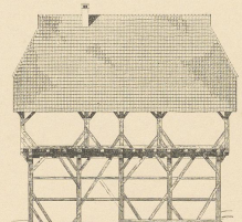
Abb. 9. Längsschnitt. Ursprünglicher Zustand.
