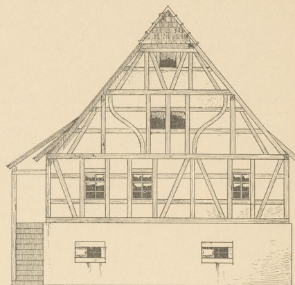
Abb. 2. Hinteransicht des Wirtschaftshauses.
