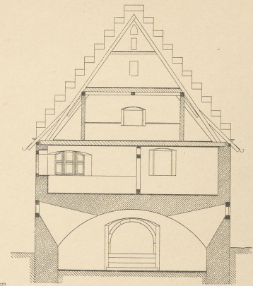
Abb. 3. Schnitt AB.
