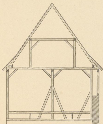
Abb. 5. Querschnitt der Scheune.
