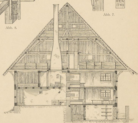
Abb. 4. Querschnitt A B.
