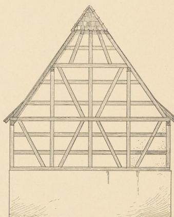
Abb. 6. Giebelansicht der Scheune.
