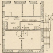
Abb. 6. Grundriss des Wohnhauses.
