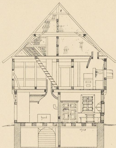
Abb. 3. Kippenheim Nr. 227. Querschnitt. Massstab zu Abb. 3, 5, 6, 8 und 11.
