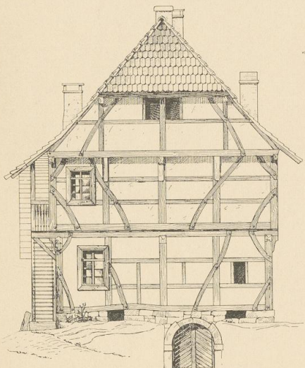
Abb. 5. Kippenheim Nr. 227. Vordergiebel.
