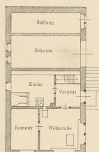
Abb. 5. Herbolzheim. Hauptgeschoss.
