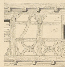
Abb. 10. Herbolzheim. Detail der Front.
