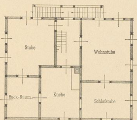
Abb. 9. Wohngeschoss des Wirtschaftshauses.
