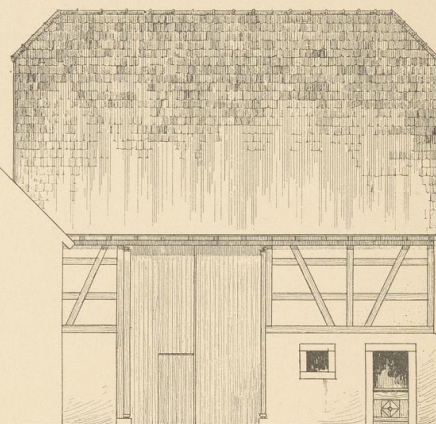
Abb. 4. Ansicht der Scheune mit Stall.
