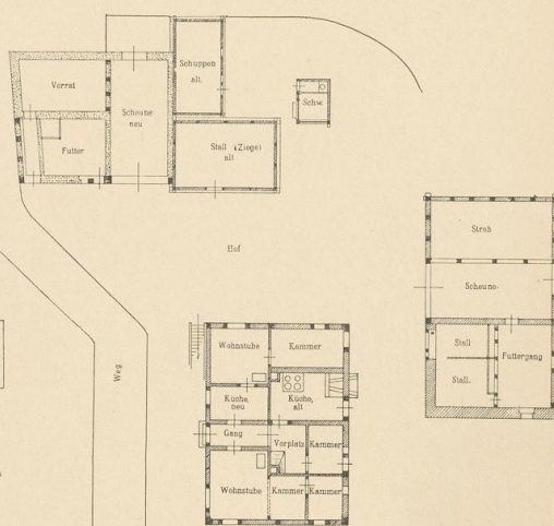
Abb. 13. Kippenheim Nr. 227. Gehöftgrundriss.
