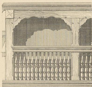
Abb. 1. Kippenheim Nr. 58. Holzlaube.
