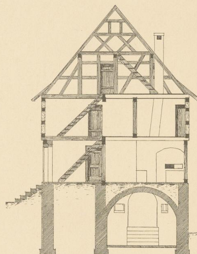
Abb. 4. Querschnitt.
