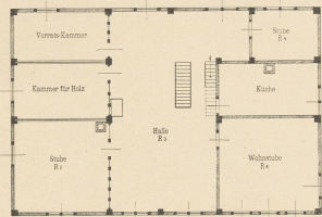
Abb. 5. Grundriss des Obergeschosses.
