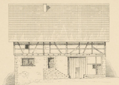
Abb. 2. Herbolzheim. Seitenfront.
