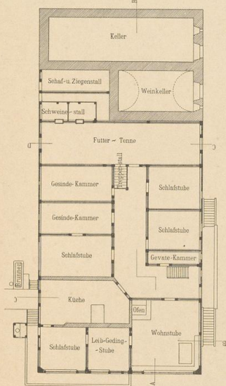
Abb. 4. Grundriss.
