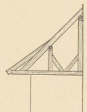
Abb. 8. Seitenansicht.
