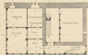
Abb. 6. Grundriss des Erdgeschosses.
