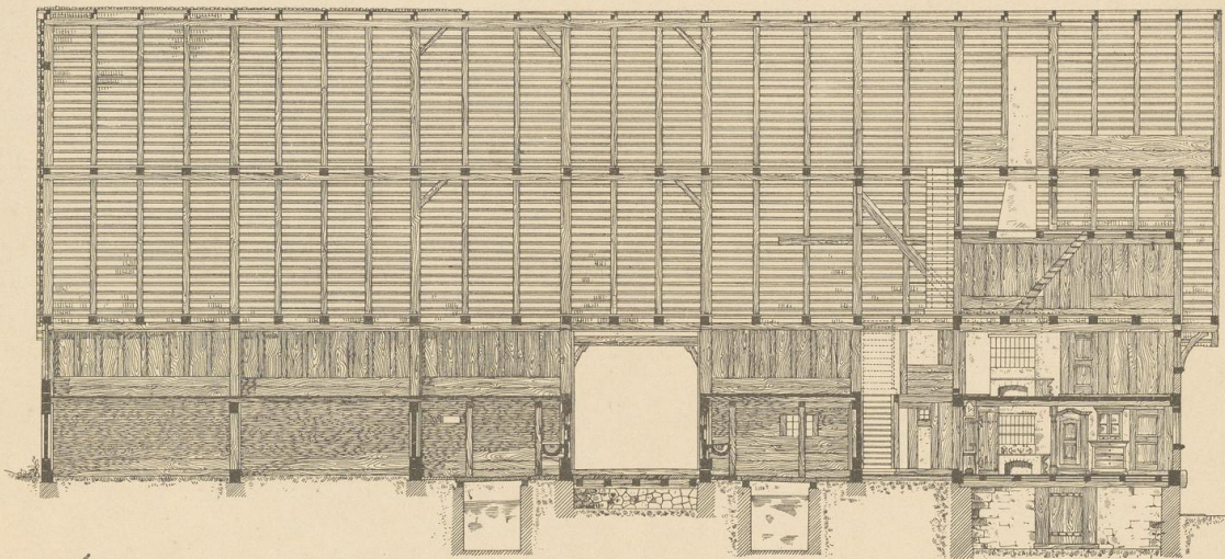
Abb. 2. Längschnitt.
