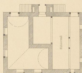
Abb. 11. Kellergeschoss des Wirtschaftshauses.
