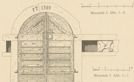
Abb. 8. Kellerthür.
