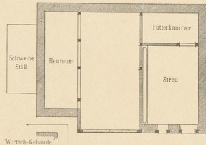
Abb. 10. Grundriss der Scheune.
