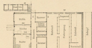
Abb. 10. Grundriss.
