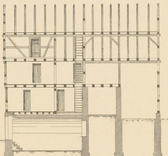
Abb. 3. Längenschnitt.
