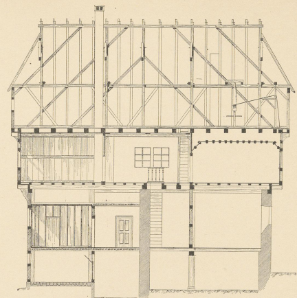
Abb. 3. Längsschnitt C D.
