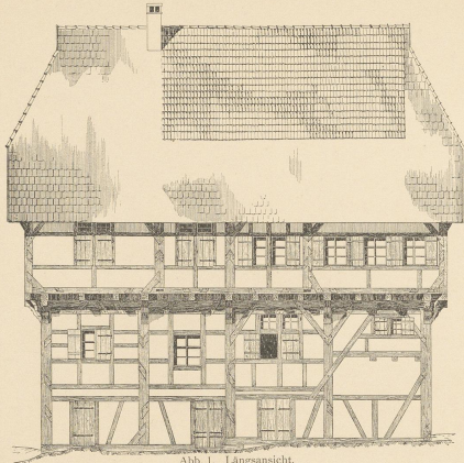
Abb. 1. Längsansicht.
