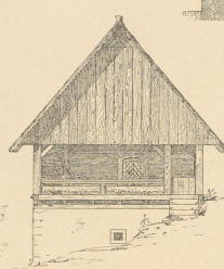
Abb. 9. Giebelansicht. Zu Abb. 10.
