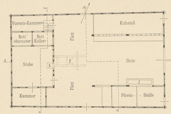
Abb. 1. Grundriss. x Ofen y Feuerstelle z Krippe.
