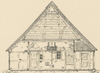
Abb. 5. Querschnitt a b.
