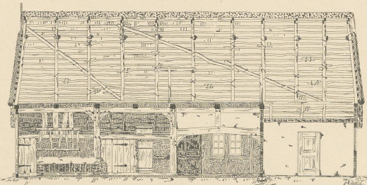
Abb. 6. Längenschnitt c d.
