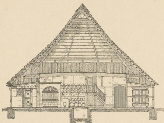
Abb. 1. Nr. 218. Schnitt A-B.
