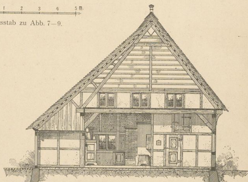
Abb. 9. Nr. 120. Schnitt A-B.
