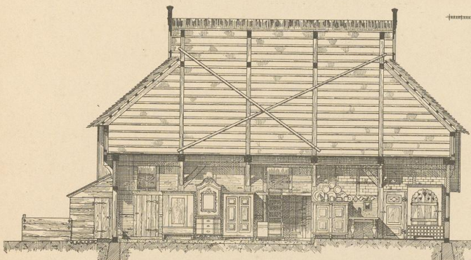
Abb. 8. Nr. 120. Schnitt C-D.
