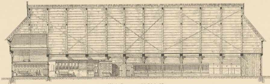
Abb. 1. Neuengamme 216, Schnitt C D.
