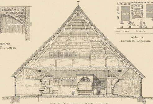
Abb. 3. Neuengamme 216, Schnitt A B.
