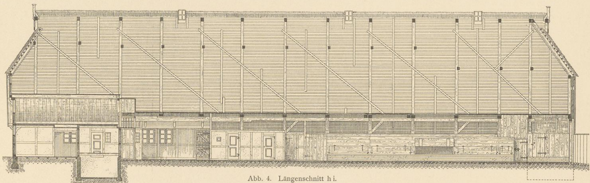
Abb. 4. Längenschnitt h i.
