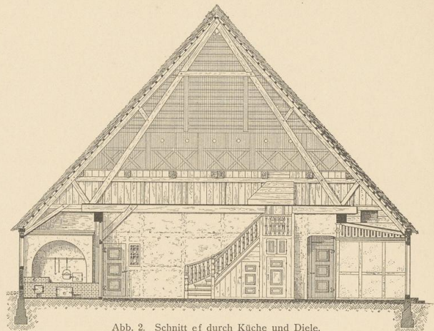
Abb. 2. Schnitt ef durch Küche und Diele.
