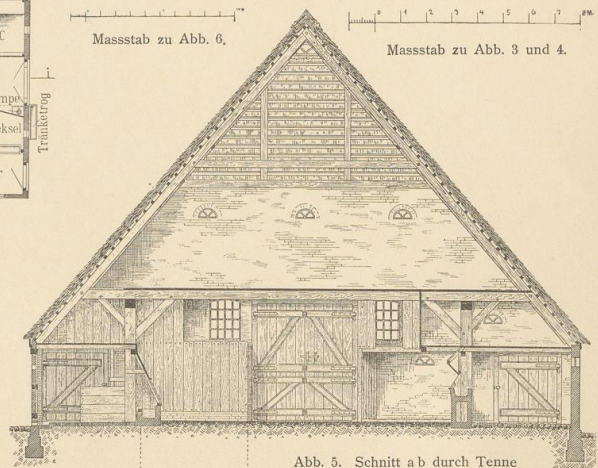
Abb. 5. Schnitt ab durch Tenne und Ställe.
