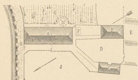
Abb. 7. Lageplan.
