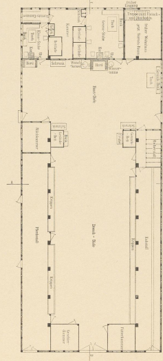
Abb. 4. Neuengamme 216, Grundriss.
