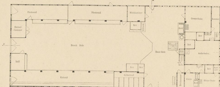
Abb. 3. Nr. 218. Grundriss.
