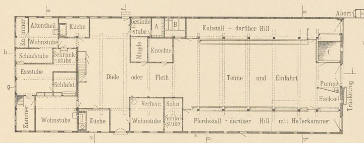
Abb. 6. Grundriss.
