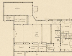
Abb. 8. Lamstedt, Grundriss.
