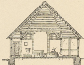
Abb. 7. Lamstedt, Schnitt A B.
