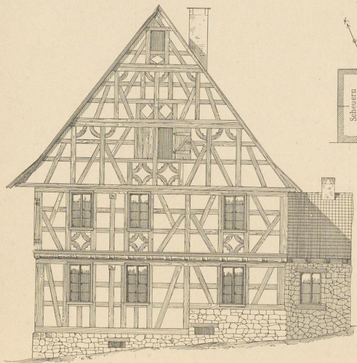
Abb. 2. Giebelansicht.
