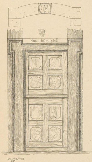
Abb. 7. Hausthür.
