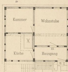
Abb. 9. Erdgeschoss vom „Bau“.
