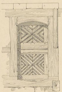
Abb. 13. Hausthür n in Abb. 9. 1:40.
