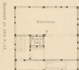
Abb. 11. Obergeschoss vom „Bau“.
