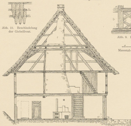
Abb. 2. Querschnitt CD.
