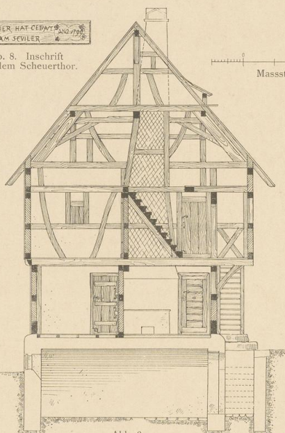
Abb. 3. Der „Bau“ B, Schnitt nach a b.
