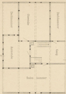
Abb. 4. Dachgeschoss des Wohnhauses.
