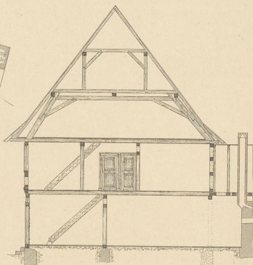
Abb. 3. Querschnitt.
