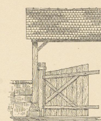
Abb. 5. Rückansicht.
