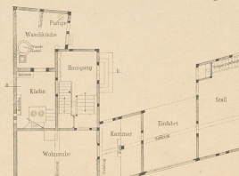
Abb. 8. Untergeschoss des Wohnhauses.
