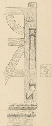
Abb. 8. Eckpfosten.
