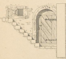
Abb. 14. Kellereingang beim „Bau“.
