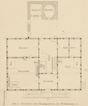
Abb. 5. Grundriss vom Hauptgeschoss des Wohnhauses A.
