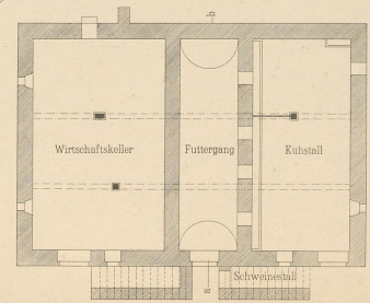
Abb. 6. Kellergeschoss des Wohnhauses.
