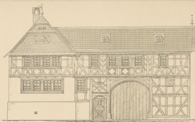
Abb. 2. Ansicht nach der Strasse.
