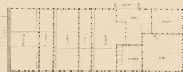
Abb. 5. Grundriss vom unteren Stock.
