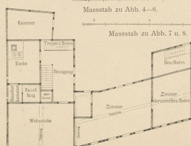
Abb. 7. Obergeschoss des Wohnhauses.
