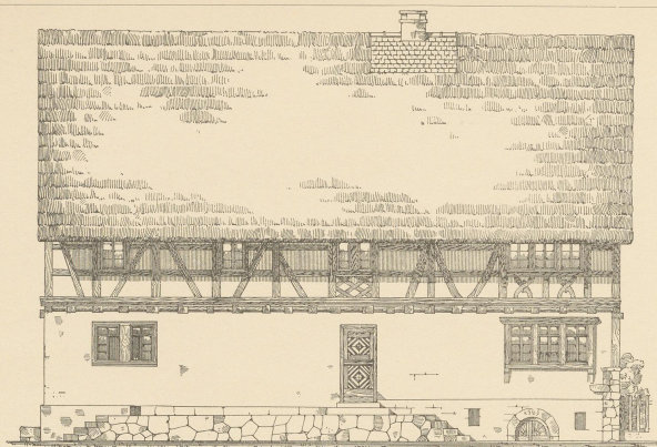
Abb. 1. Längsansicht.
