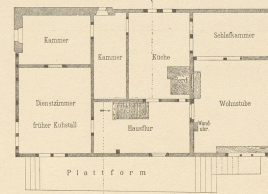
Abb. 12. Erdgeschoss.
