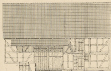
Abb. 4. Ansicht der Scheune.
