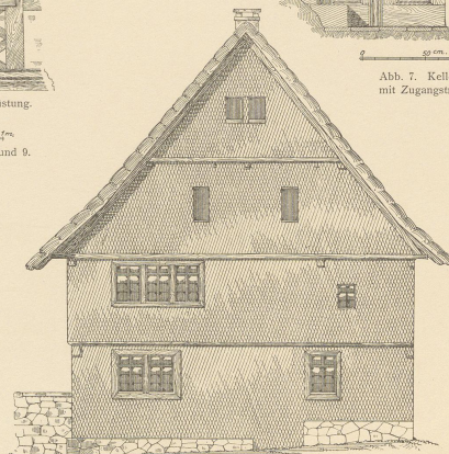
Abb. 3. Giebelansicht.
