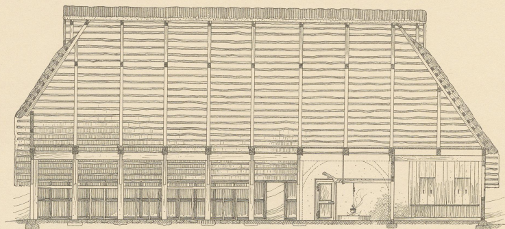
Abb. 3. Mansholt. Längenschnitt a b.
