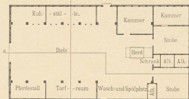
Abb. 6. Mansholt. Grundriss.
