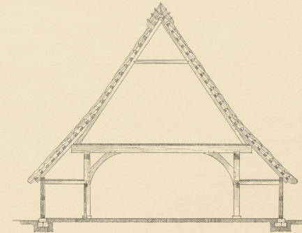
Abb. 4. Mansholt. Querschnitt c d.
