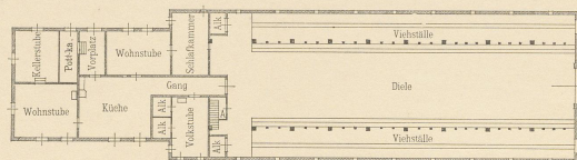
Abb. 5. Osterseefeld. Grundriss.
