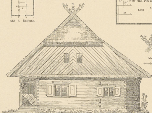
Abb. 4. Wohnhaus, Giebelseite.
