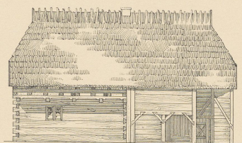
Abb. 6. Längensicht. Strassenseite.
