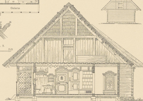
Abb. 5. Wohnhaus, Querschnitt.
