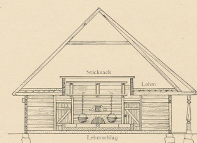
Abb. 9. Querschnitt.
