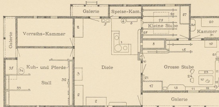
Abb. 1. Wohnhaus, Erdgeschoss.
