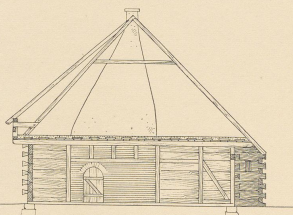
Abb. 7. Querschnitt a b.
