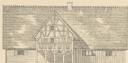
Abb. 3. Wohnhaus zum Gehöft eines Grossbauern in Ebersbach bei Braunsberg.
