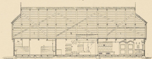
Abb. 3. Wohnhaus, Längenschnitt.
