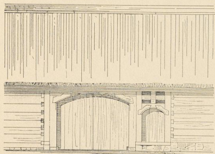
Abb. 11. Ansicht. 1:100.
