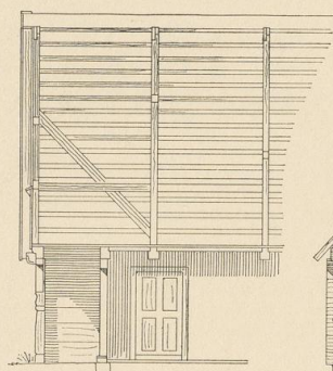
Abb. 2. Schnitt durch den Giebel.
