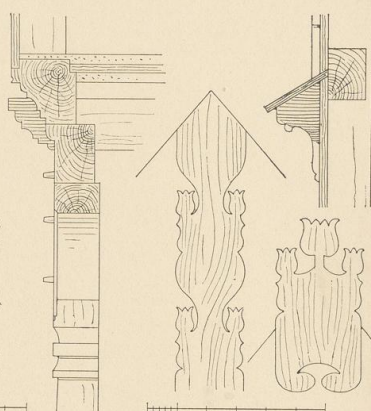
Abb. 10. Vom Giebel. 1:15.
