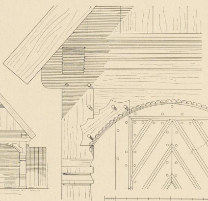
Abb. 9. Linke Ecke der Halle. 1:20.
