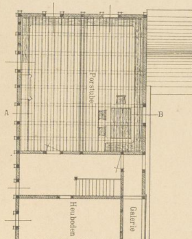
Abb. 4. Monstab. Grundriss vom Obergeschoss.
