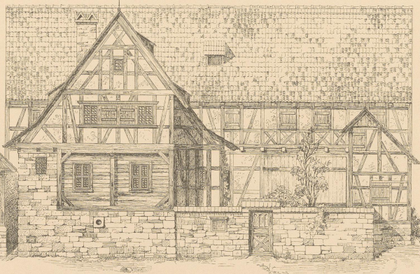
Abb. 2. Strassen-Ansicht.
