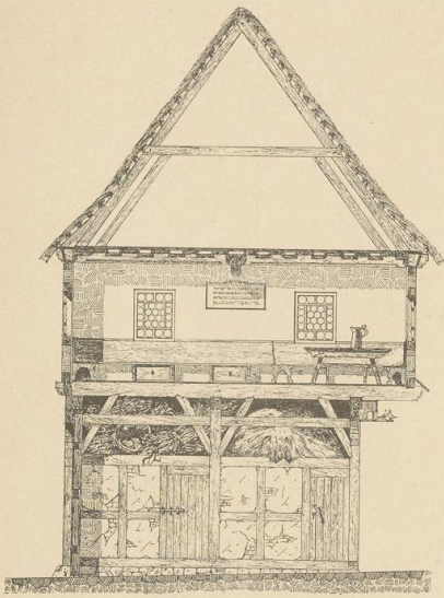
Abb. 1. Thorgebäude mit Porstube in Monstab. Querschnitt AB.
