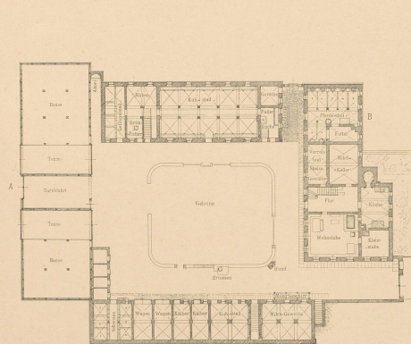
Abb. 3. Grundriss vom Erdgeschoss.
