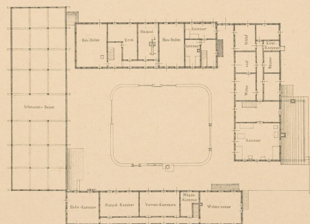
Abb. 4. Grundriss vom Obergeschoss.
