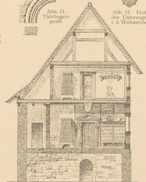
Abb. 3. Querschnitt.
