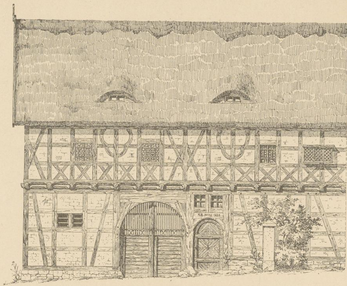
Abb. 2. Thorgebäude mit Porstube in Monstab. Ansicht an der Dorfstrasse.
