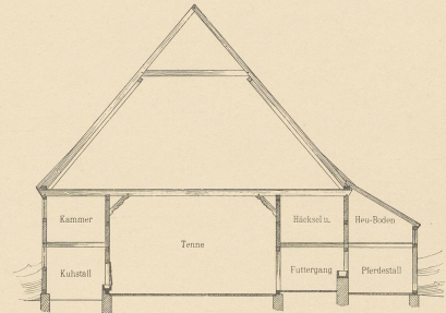
Abb. 4. Querschnitt.
