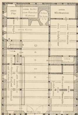
Abb. 10. Haus Schupers, Grundriss.
