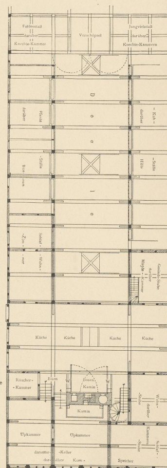
Abb. 3. Bispinghof, Grundriss.
