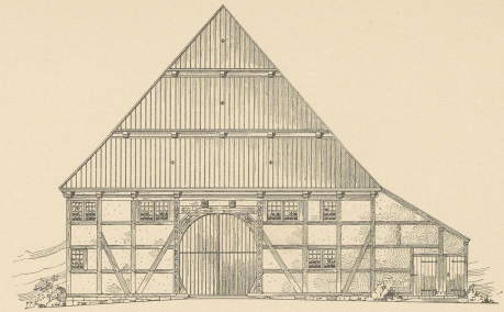
Abb. 2. Giebelansicht.
