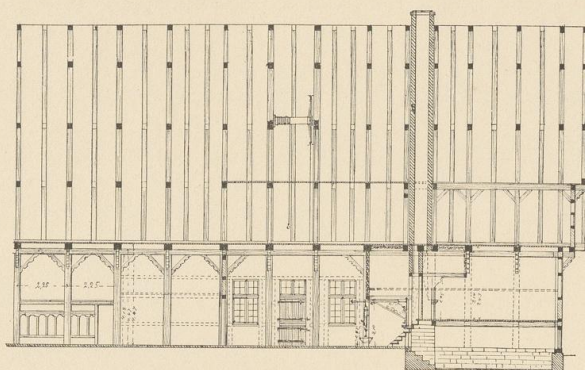
Abb. 1. Bispinghof, Längenschnitt.
