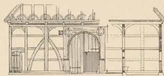
Abb. 5. Doppelhaus in Bödexen. Strassenansicht. Schnitt. Meiners und Grote Kreis Höxter.
