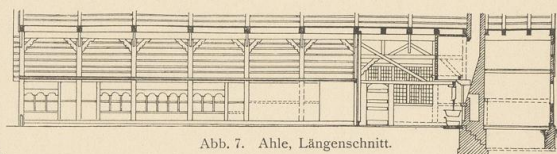
Abb. 7. Ahle, Längenschnitt.
