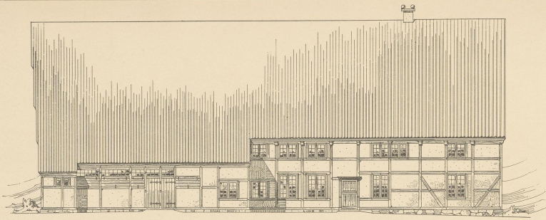
Abb. 1. Längsansicht.
