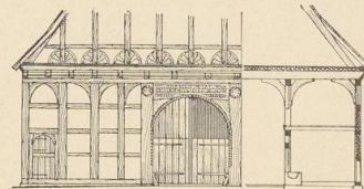
Abb. 10. Valepagothof. Giebelansicht. Querschnitt.
