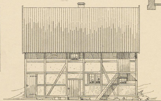
Abb. 6. Backhaus.
