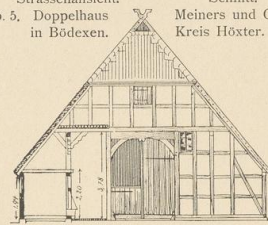
Abb. 6. Bauernhaus in Rahden, Kreis Lübbecke. Querschnitt. Südansicht.
