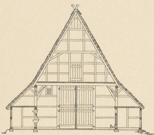
Abb. 4. Ahle, Querschnitt durch die Deele.
