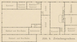
Abb. 8. Zwischengeschoss.
