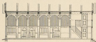
Abb. 2. Haus Warneke in Bödexen. Längsschnitt.
