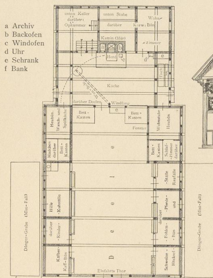
Abb. 8. Ahle, Grundriss.
