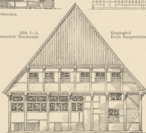
Abb. 2. Bispinghof, Nordostgiebel.
