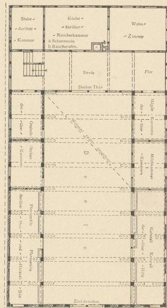
Abb. 11. Valepagothof. Grundriss.
