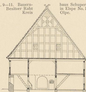
Abb. 11. Haus Schupers, Querschnitt.
