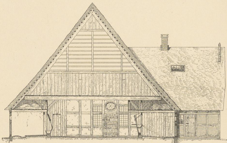
Abb. 3. Querschnitt durch Diele und Ställe.
