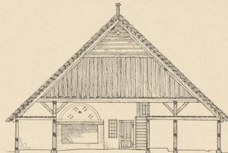
Abb. 3. Haus Schlappkohl, Querschnitt.
