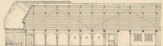
Abb. 4. Haus Axen in Lindholm. Längenschnitt.
