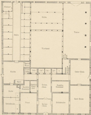
Abb. 3. Rother Hauberg. Grundriss.
