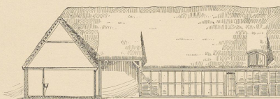
Abb. 9. Wonsbeck. Hofansicht der Scheune mit Schnitt durch den Pferdestall.
