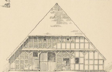
Abb. 19. Scheune in Gollendorf. Giebelansicht.
