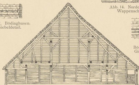
Abb. 13. Haus Dyrsen in Norderdeich. Querschnitt e d.
