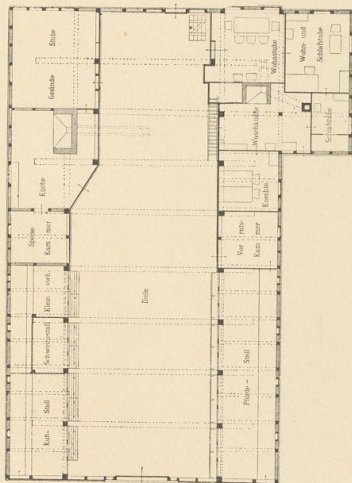
Abb. 4. Grundriss.
