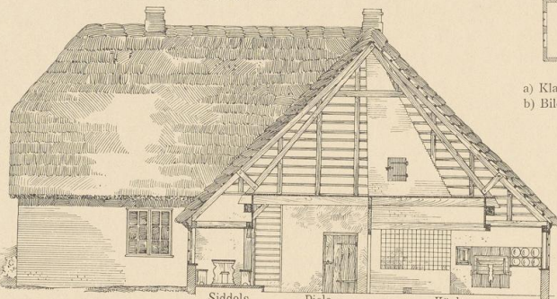
Abb. 2. Haus Groth in Bödinghusen. Querschnitt x y.
