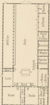
Abb. 10. Haus Hinrich Rix in Schönbeck. Grundriss.
