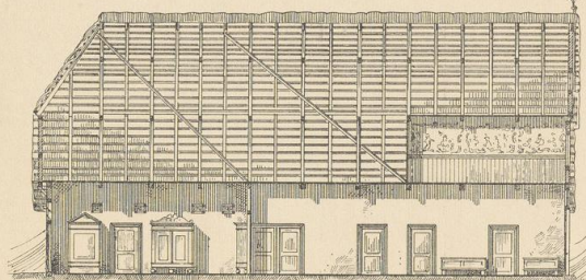
Abb. 4. Haus Petersen in Blieschendorf. Längenschnitt.
