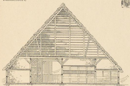
Abb. 18. Scheune in Gollendorf. Querschnitt.
