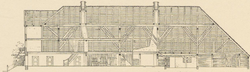
Abb. 13. Hochdorfer Hauberg. Längenschnitt.
