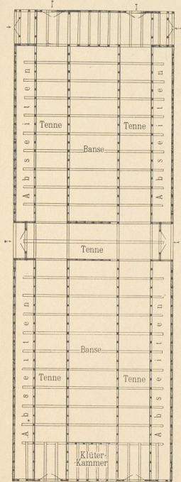
Abb. 15. Scheune auf Gut Hagen i. d. Probstei. 1:600.
