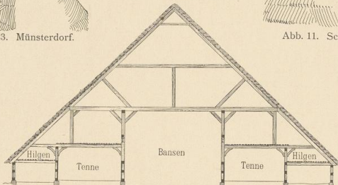
Abb. 13. Scheune auf Gut Hagen. Querschnitt.
