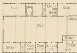
Abb. 24. Haus Makeprang in Dänschendorf. Erdgeschoss.
