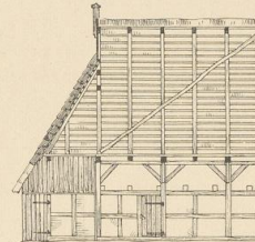
Abb. 5. Haus Schlappkohl. Längenschnitt.
