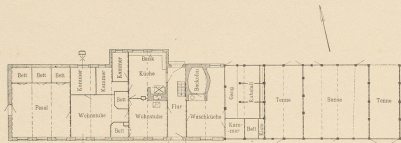
Abb. 2. Bauernhaus auf Barsö. Grundriss.
