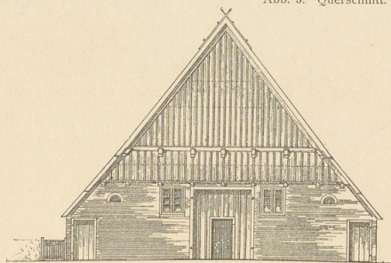
Abb. 5. Giebelansicht.
