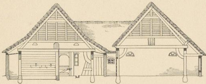
Abb. 3. Haus Axen in Lindholm. Querschnitt.
