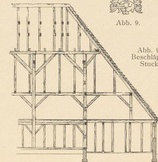
Abb. 6. Rother Hauberg. Längenschnitt.
