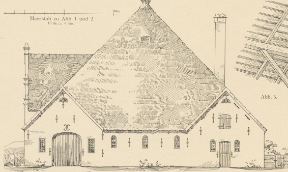
Abb. 2. Rother Hauberg. Nordansicht.
