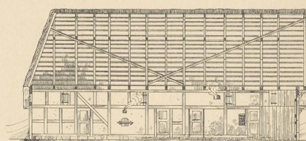
Abb. 22. Haus Makeprang in Dänschendorf. Längenschnitt.
