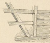
Abb. 17. Bansenwand aus der Scheune auf Gut Hagen.
