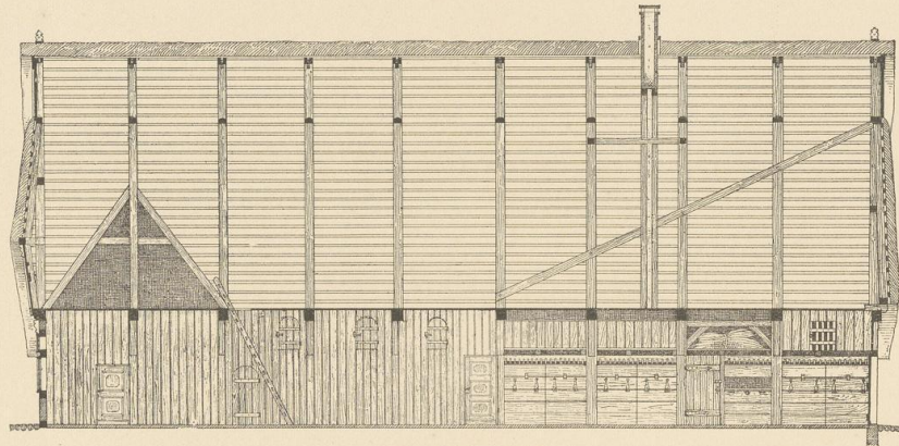
Abb. 1. Längenschnitt.
