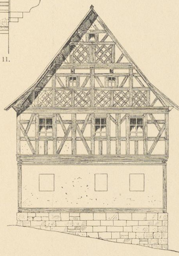
Abb. 4. Bauernhaus No. 35 aus Mönchröden, Giebelseite.
