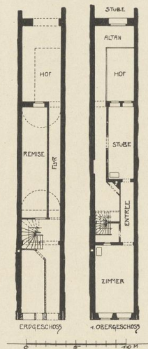
Abb. 20 u. 21. Wohnhaus Ring No. 54. (G.)
