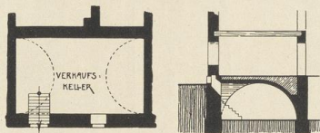
Abb. 28. Herrenstr. No. 14. (G.)
