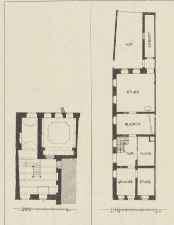
Abb. 36. Wohnhaus. Neue Weltgasse No. 34. Erdgeschoss. (G.)
