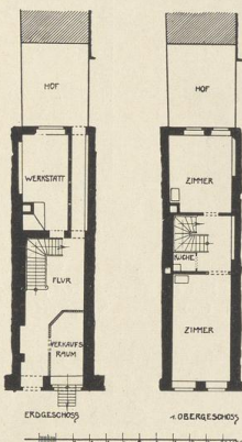
Abb. 22 u. 23. Haus Schmiedebrücke No. 15. (G.)
