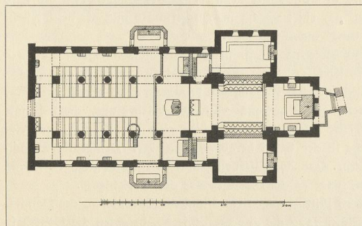
Abb. 1. Kloster Wiblingen. Grundriss der alten romanischen Kirche. (G.)
