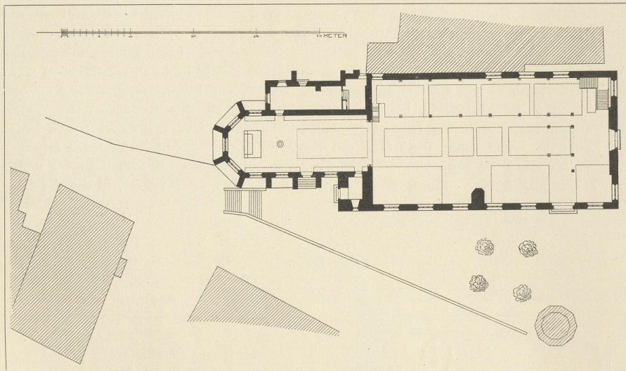
Abb. 5. Grundriss der Prediger- (Spital-) Kirche. (St.)
