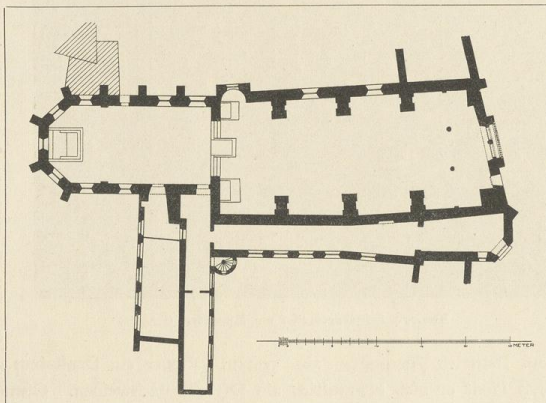
Abb. 6. Grundriss der Mengenlosterkirche. (St.)
