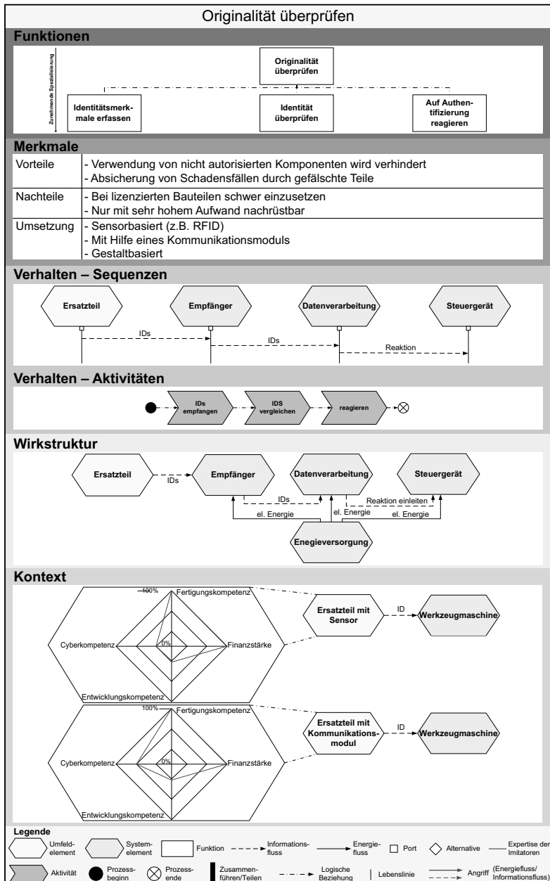
Bild A-20: Schutzmuster Originalität überprüfen
