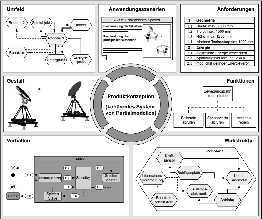
Bild 3-8: Partialmodelle zur Beschreibung des Systemmodells [DGO+14, S.38]
