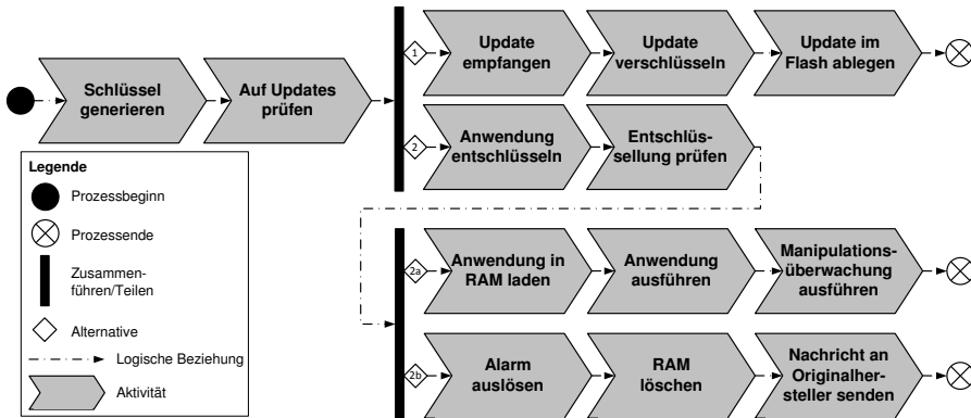
Bild 4-5: Verhaltensmodell der Schutzmaßnahme Protecting Electronic Products
