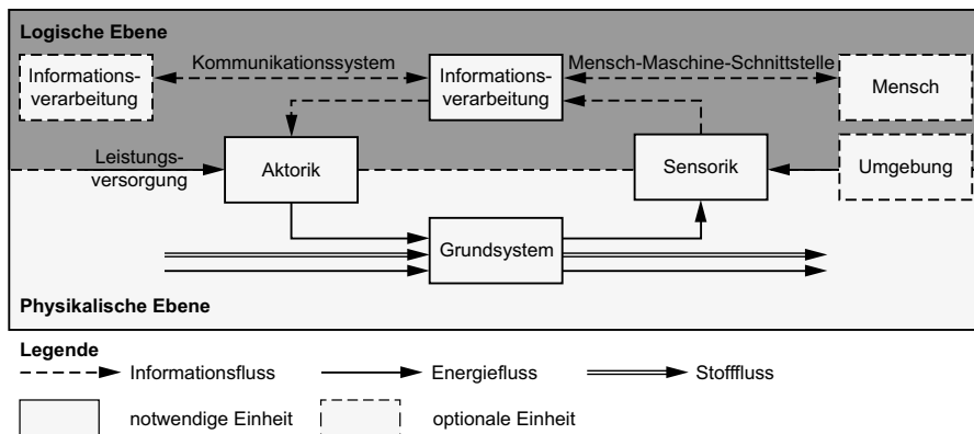
Bild 2-3: Grundstruktur eines mechatronischen Systems nach [VDI2206, S.14]
