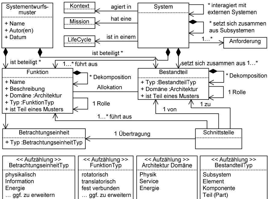
Bild 3-14: Metamodell für ein lösungsmusterbasiertes Systems Engineering nach PFISTER (vgl. [PCH+11])
