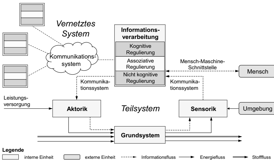
Bild 2-5: Technologiekonzept Intelligenter Technischer Systeme [GTD13]
