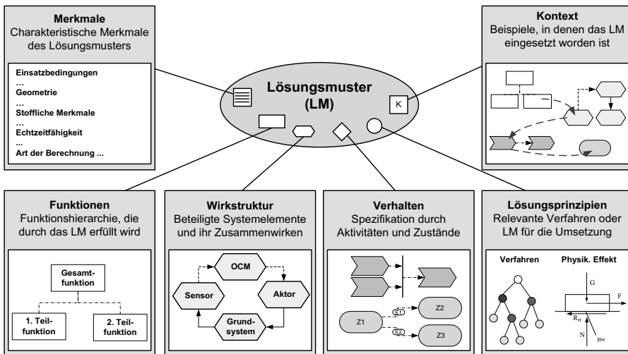
Bild 3-10: Spezifikation eines Lösungsmusters nach DUMITRESCU [Dum10, S.130]
