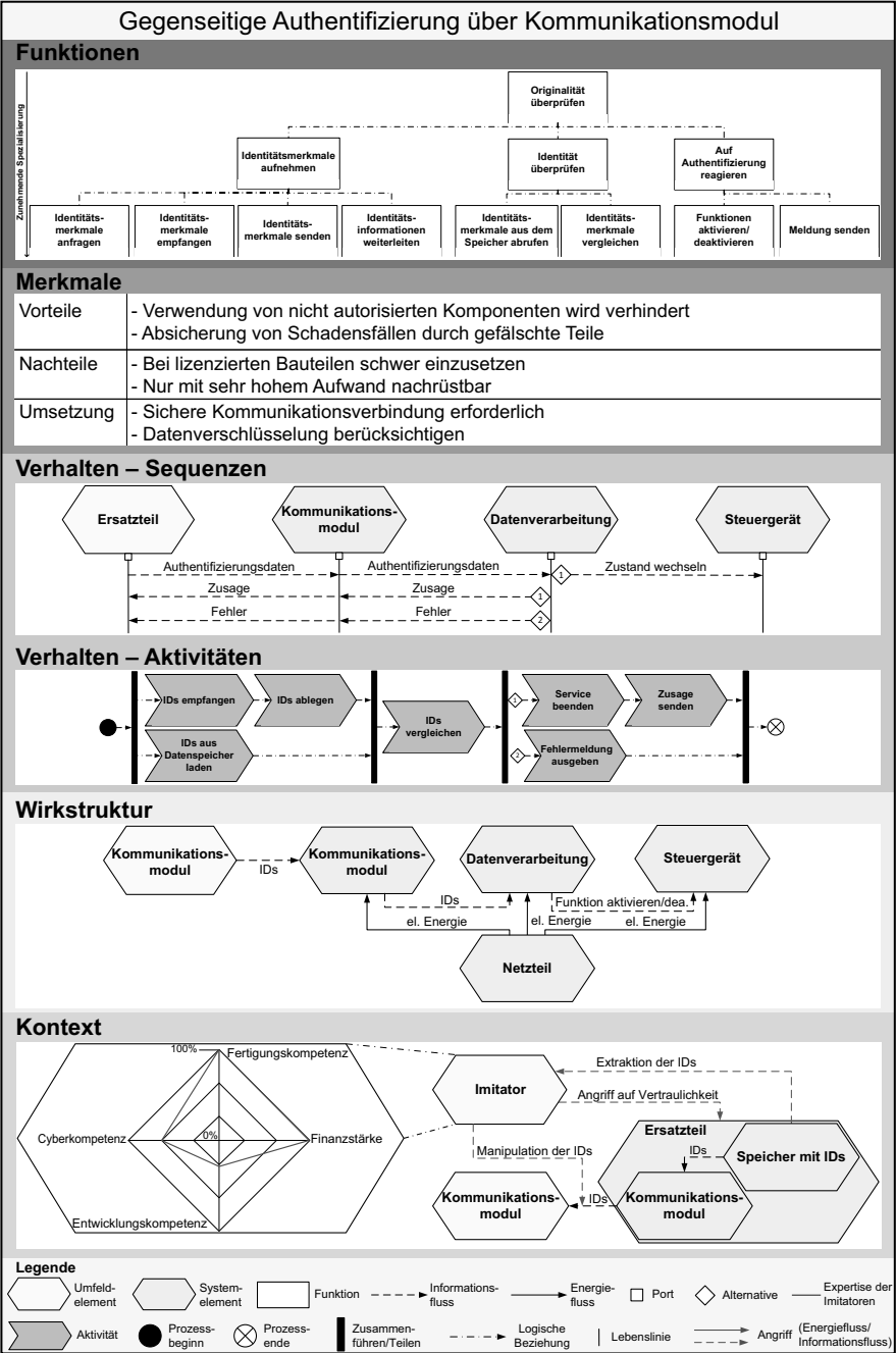
Bild A-22: Schutzmuster gegenseitige Authentifizierung über Kommunikationsmodul
