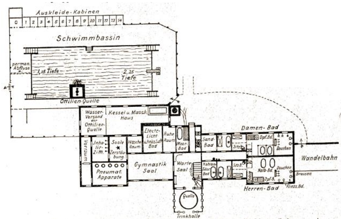
Abb. 9: Grundriss Badehaus, 1903
