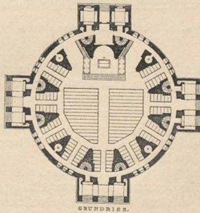
Abb. 75. Vierter Entwurf zu einer Kirche für die Dranienburger Vorstadt in Berlin. Grundriß. 1828.
