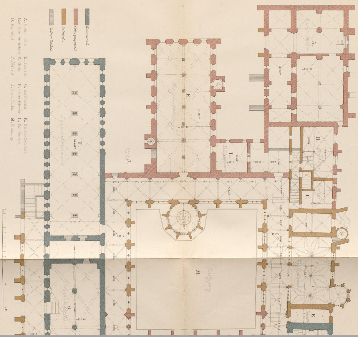
Grundriss der Cisterzienser-Abtei Maulbronn.
