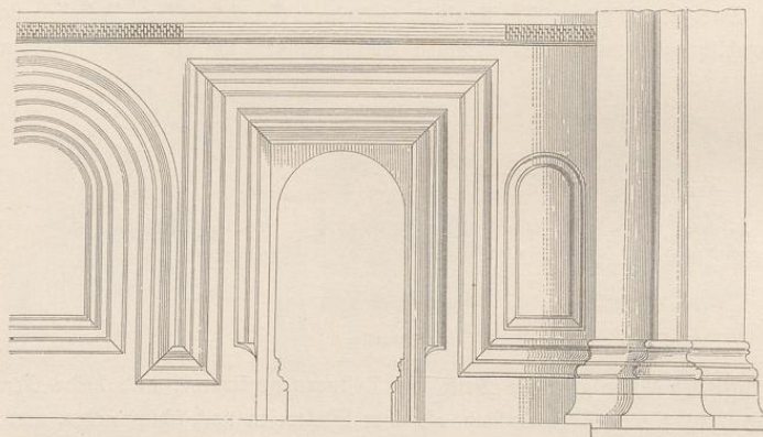
Ansicht des Letzners vom Chor aus. \frac{1}{50} nat. Größe.
