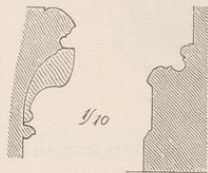
Profile vom Westflügel des Kreuzgangs.
