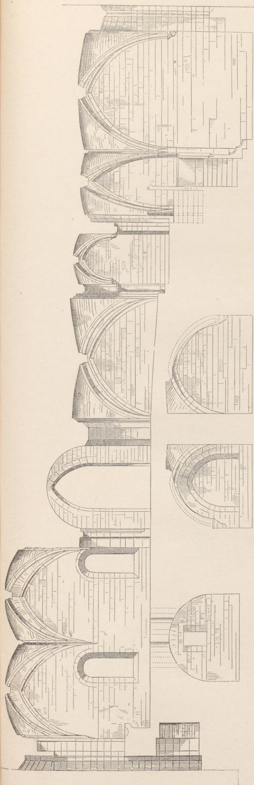
Schnitt durch die Wärmehalle bis zur Bundeshalle. 1/100 nat. Größe.
