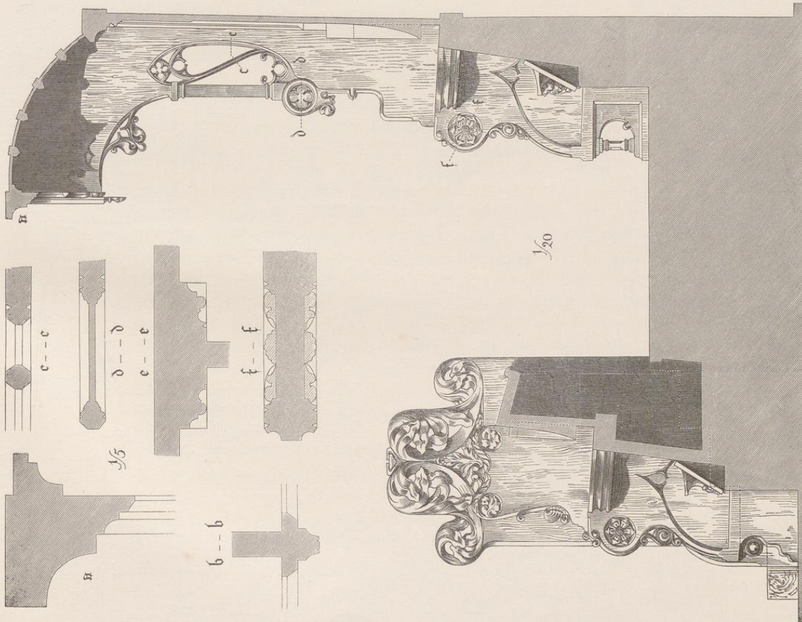
Querschnitt und Anlauf der Chorflügel. \frac{1}{20} nat. Größe.
