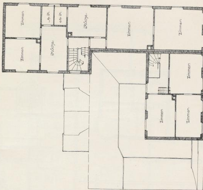
Obergeschoss-Grundriss
