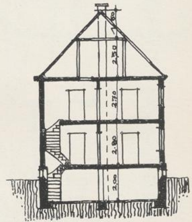
SCHNITT A-B.
