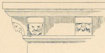
Fig. 238. Roman. Franz. Konsolengesimse.
