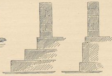
Fig. 127. Fundamentverbreiterung.
