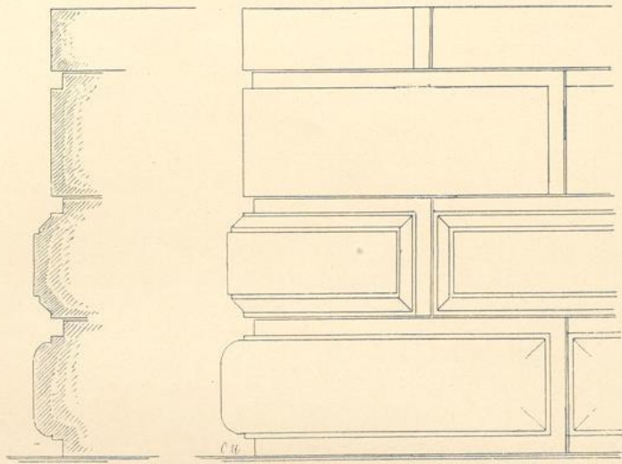
Fig. 196. Römischer Quaderverband.
