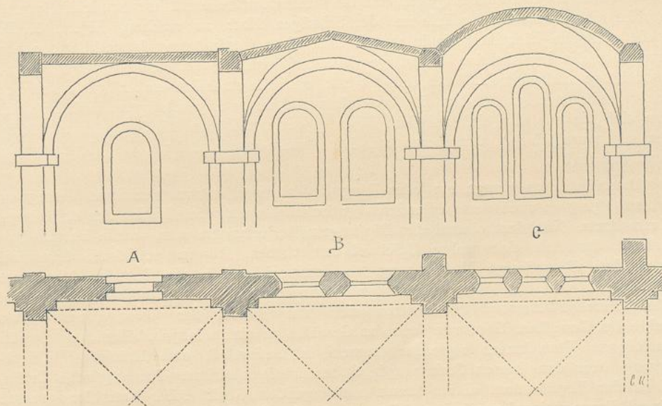
Fig. 145. Kreuzgewölbe mit Quergurten.
