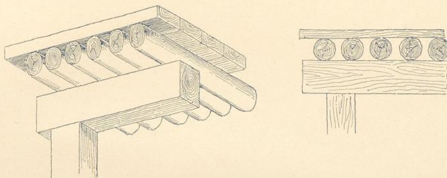
Fig. 166. Entstehung des Zahnschnitts.
