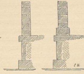
Fig. 128. Fig. 129. Bau mit Fuss und Sockel.
