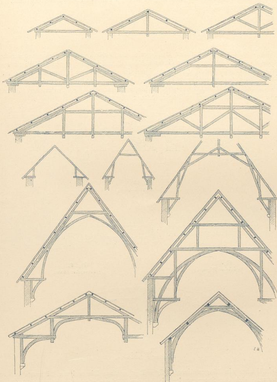
Fig. 82. Dachstuhlssysteme.
