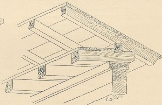
Fig. 137. Holzbalkenlage mit Dach.
