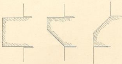
Fig. 169. Quaderschichte, nach unten oder oben abgeschrägt.
