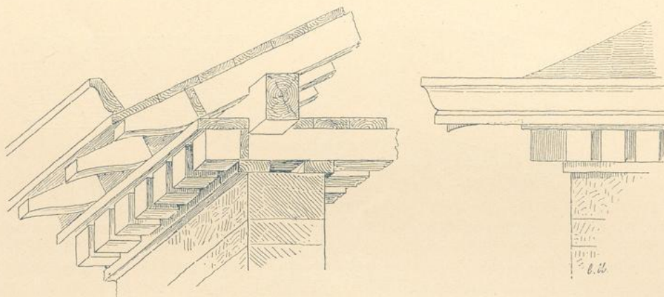
Fig. 168. Entstehung des Sparrenkopfs.
