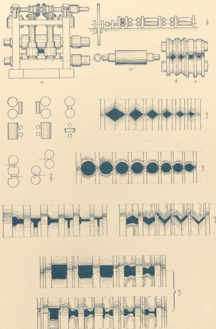
Fig. 121. Walzwerk und Façoneisen
