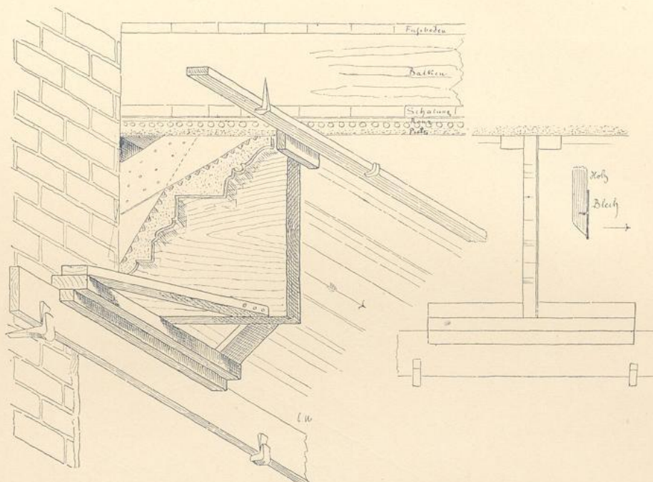
Fig. 114. Gipsziehen an Ort und Stelle.
