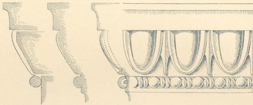
Fig. 159. Antiker Eierstab mit Schnur.
