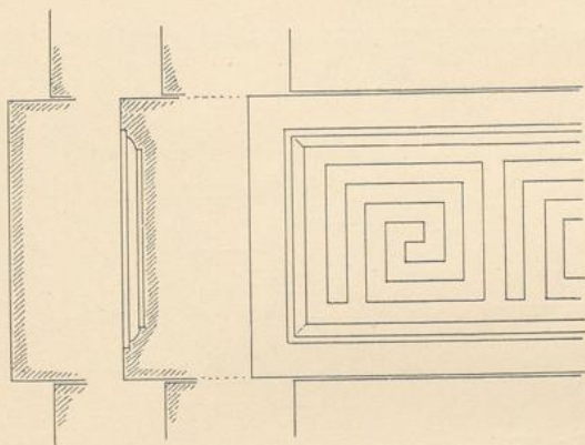
Fig. 199. Bandförmiges Gurtgesimse.
