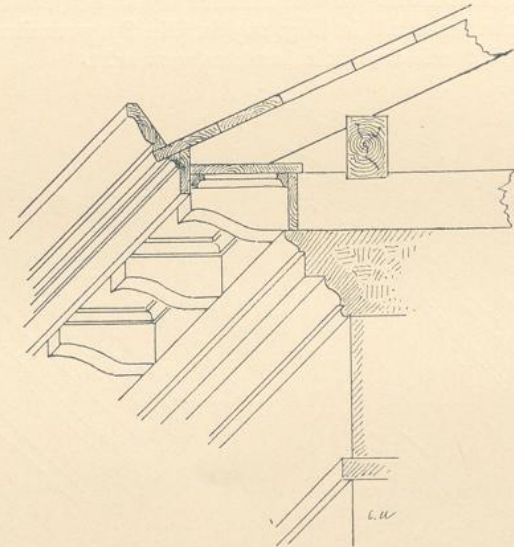
Fig. 206. Hauptgesimse mit durch- gehender Balkenlage.
