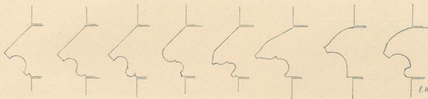
Fig. 235. Gotische Gurtgesimse XIII. bis XV. Jahrhundert.
