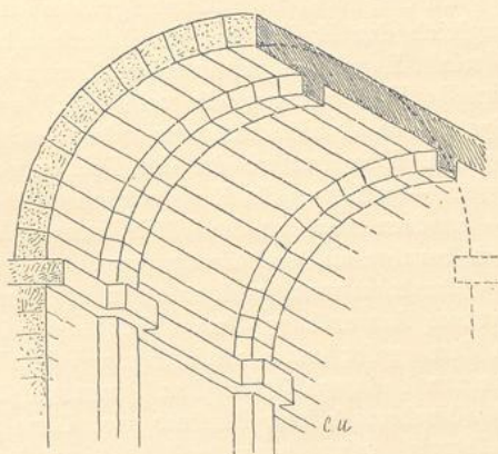
Fig. 143. Tonnengewölbe mit Quergurten.
