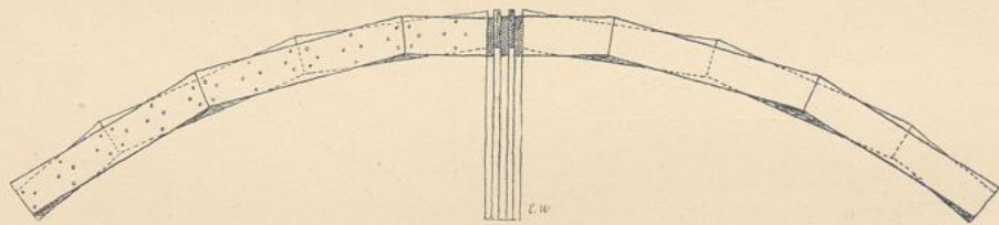
Fig. 86. Bogenförmiger Bohlenbalken.
