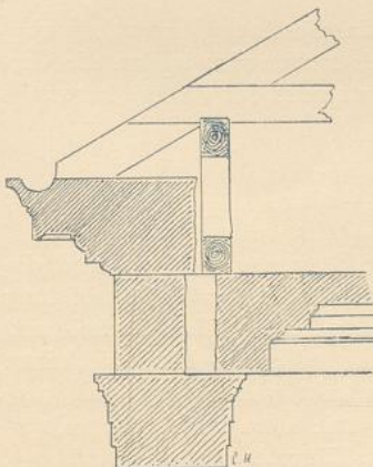
Fig. 306. Hauptgesimse mit Fries und Decken- lage im Innern.
