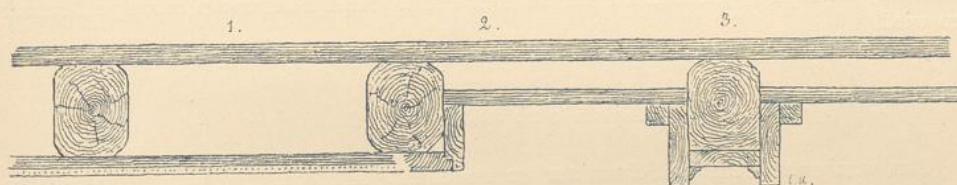
Fig. 80. Balkendecke mit Brettumkleidung.
