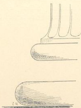
Fig. 279. Hauptglieder der Jonischen Säulenbasis.
