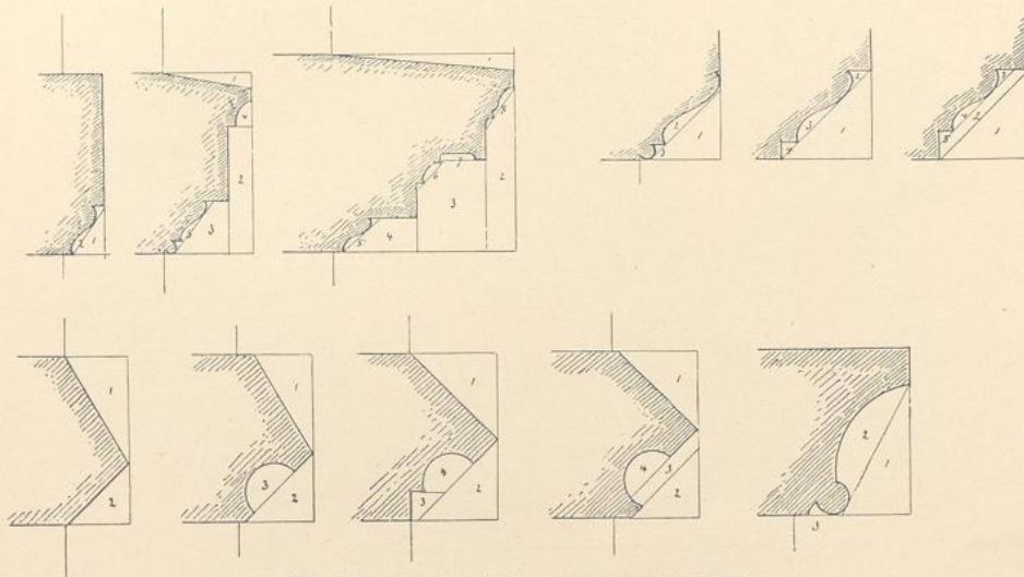
Fig. 104. Bearbeitungs-Schema verschiedener Stein-Profile.
