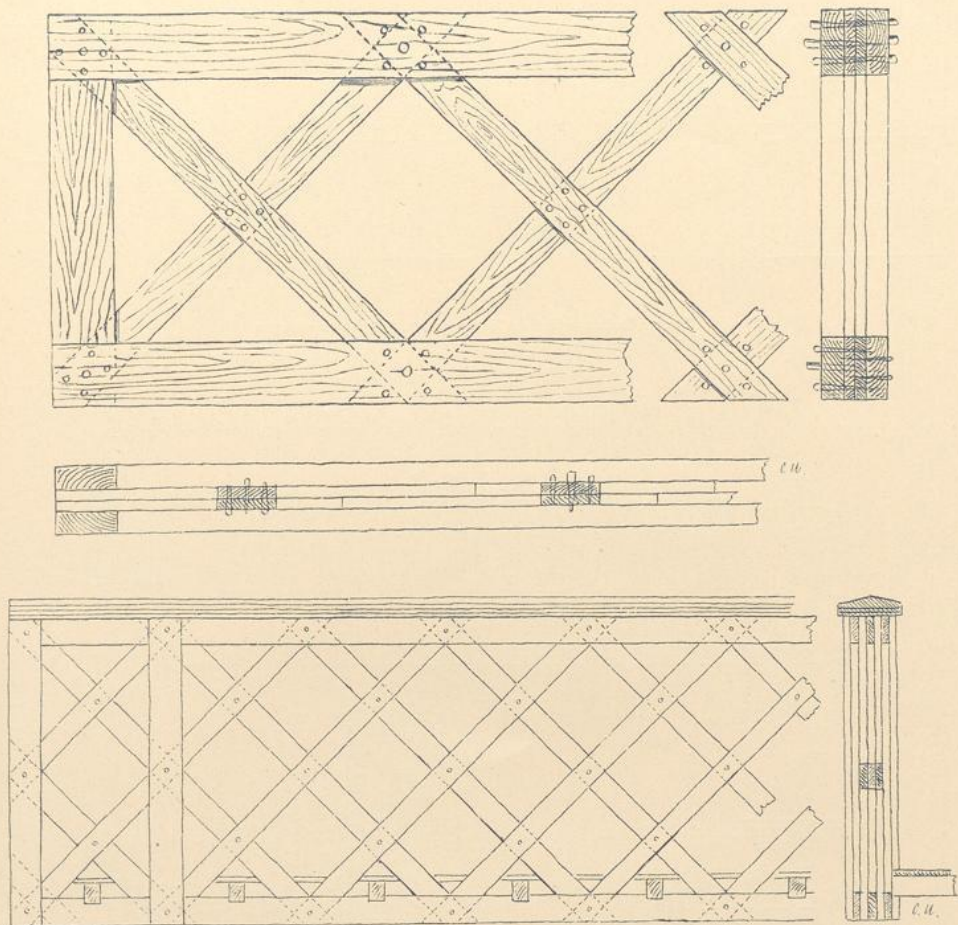
Fig. 87 und 88. Offen gebaute Gitterwerke.
