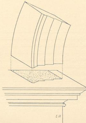
Fig. 309. Archivolte.
