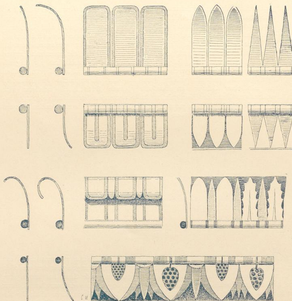
Fig. 155. Tragende Blätterreihungen.
