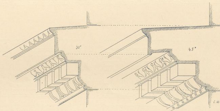
Fig. 202. Gurtgesimse mit Zahnschnitt.
