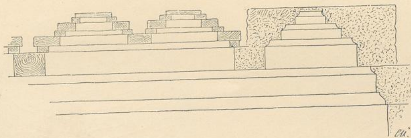
Fig. 139. Uebertragung der Holzdecke in Stein.
