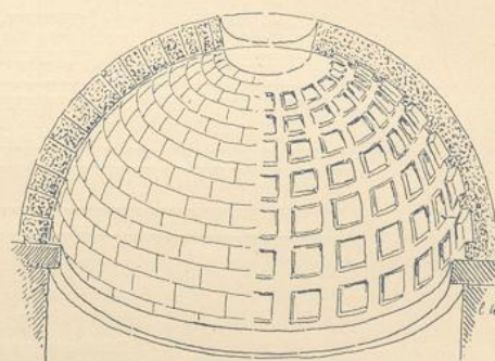
Fig. 141. Kuppel aus Quadern und kassettierte Kuppel.
