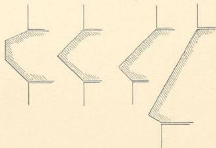
Fig. 170. Beiderseits schräg abgeschnittene Platte.
