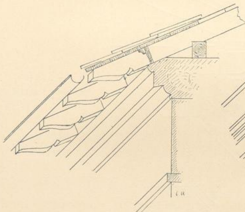
Fig. 203. Hauptgesimse mit überstehenden Dachsparren.
