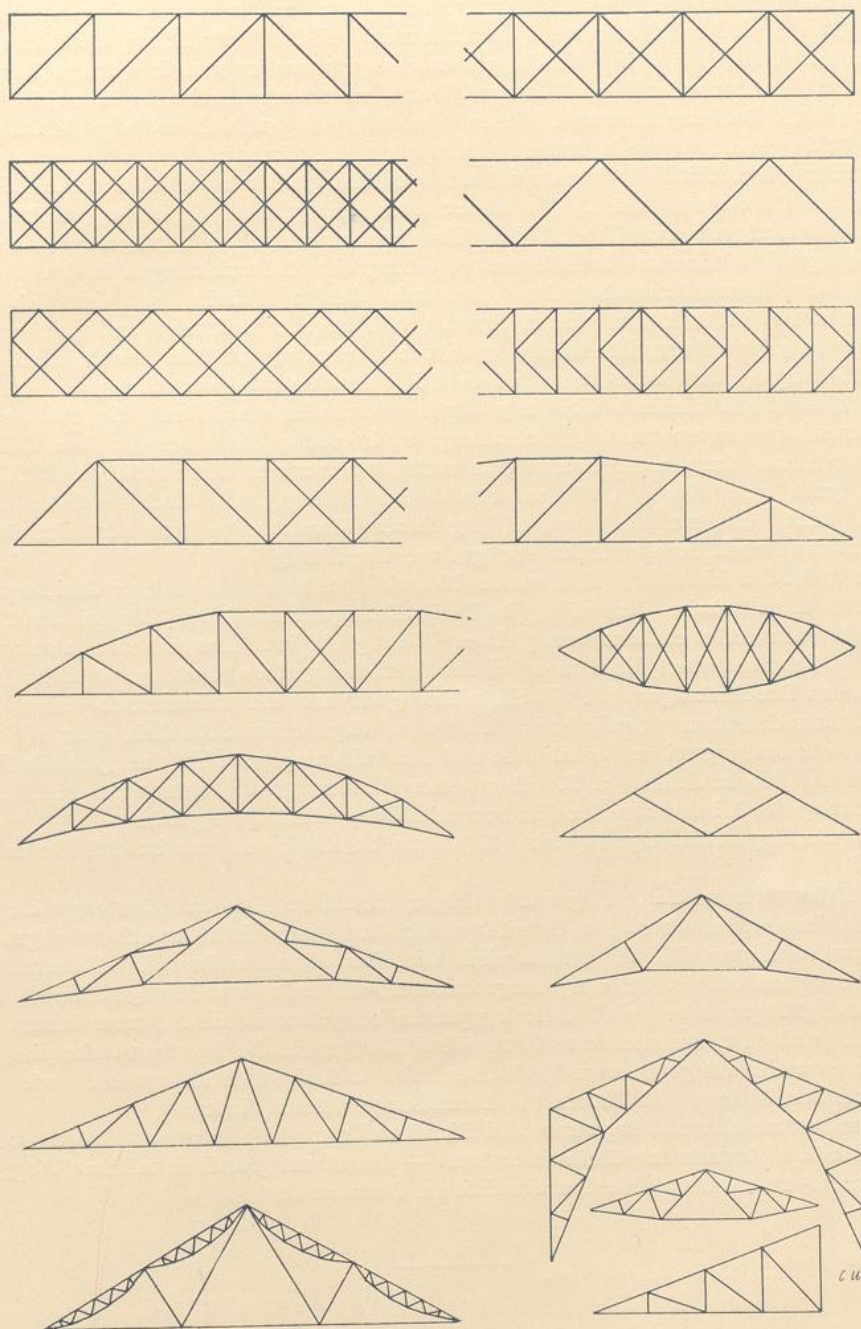
Fig. 125. Eisenträger und Dachwerke.
