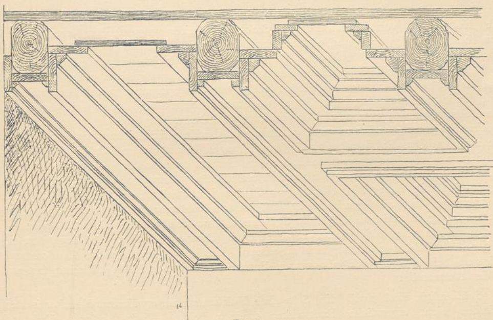
Fig. 81. Kassettendecke.
