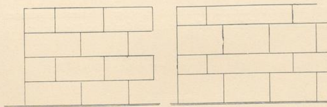
Fig. 195. Griechischer Quaderverband.
