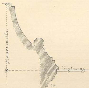
Fig. 258. Gotischer Fensterpfosten in Verbindung mit der Fensterleibung.
