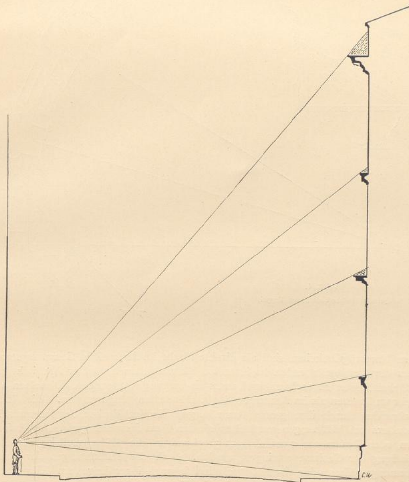
Fig. 332. Einfluss der Perspektive bezüglich der Gesimse.
