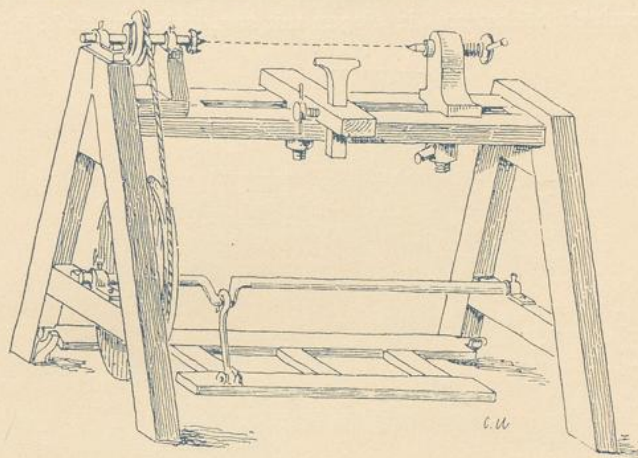
Fig. 93. Drehbank.
