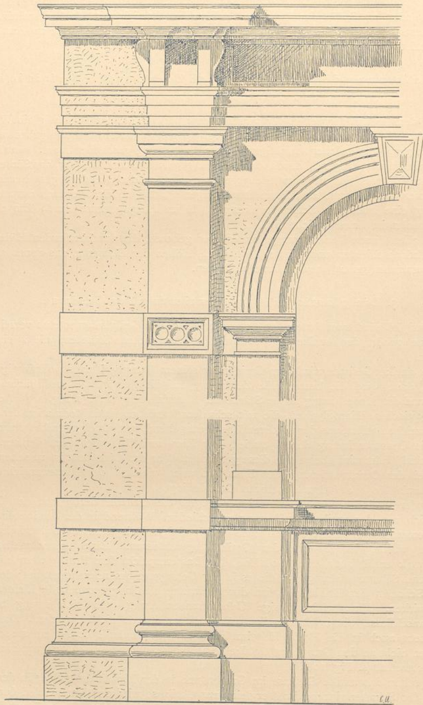
Fig. 343. Umbildung der Gesimse in einer Horizontale.
