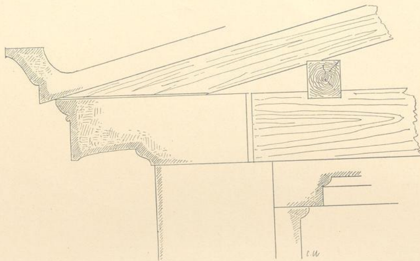
Fig. 210. Hauptgesimse v. Nike-Tempel, Athen.
