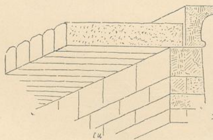
Fig. 136. Steinerne Dübeldecke.
