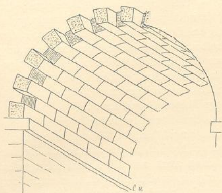
Fig. 142. Tonnengewölbe aus Quadern.
