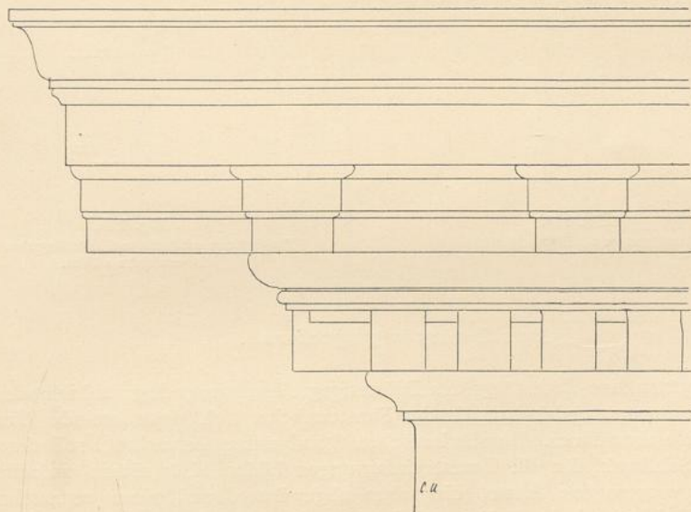
Fig. 213. Hauptgesimse mit Kastenkonsolen.
