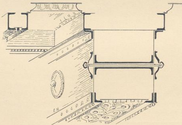
Fig. 266. Eisenarchitrav als Röhre. Herzogl. Schloss Braunschweig.
