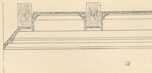
Fig. 263. Mit Brett umkleidete Balkendecke.
