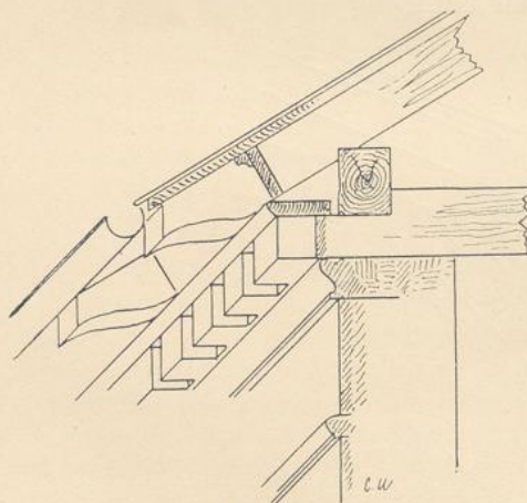
Fig. 207. Hauptgesimse mit äusserlich sichtbarer Balken- und Sparrenlage.
