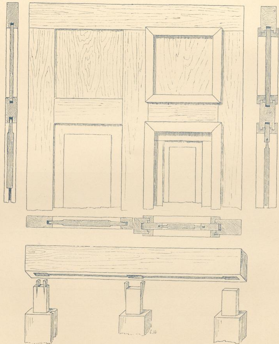
Fig. 92. Rahmenwerke aus Brett.
