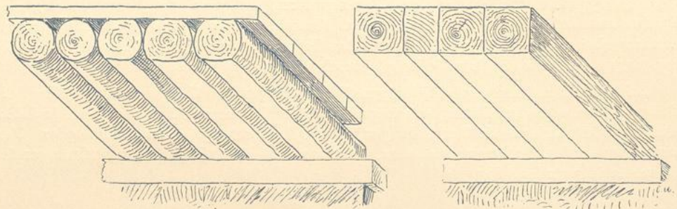
Fig. 77. Dübeldecke.
