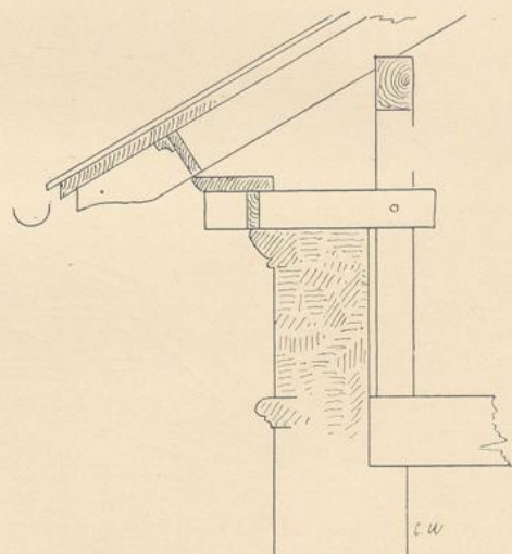
Fig. 208. Hauptgesimse mit versenkter Balkenlage.
