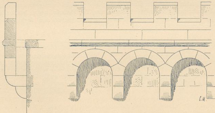
Fig. 240. Bogengesims mit Zinnen zur Verteidigung.
