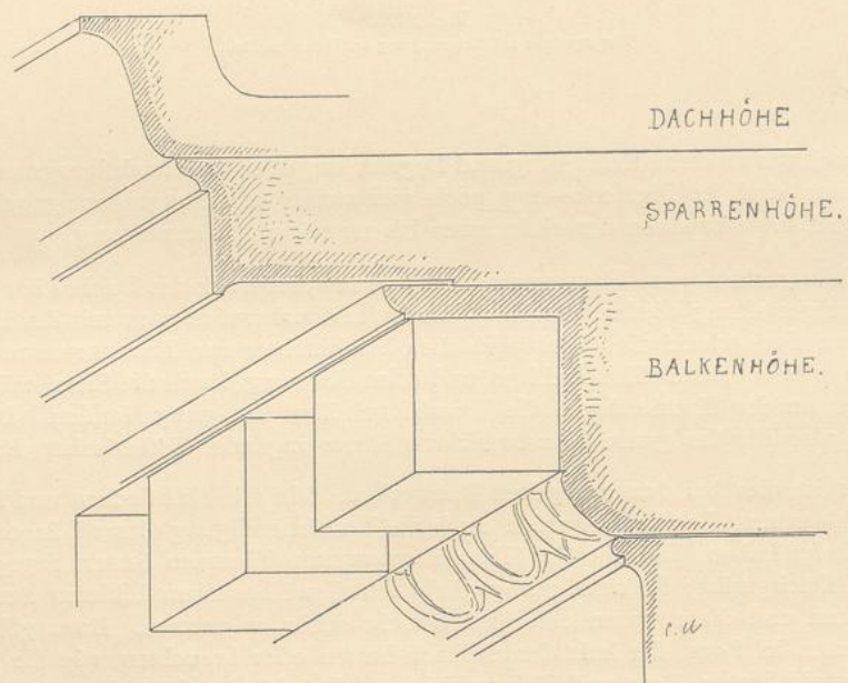
Fig. 211. Hauptgesimse v. Mausoleum, Halikarnassus.
