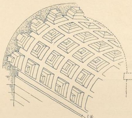
Fig. 140. Kassettierte Tonnengewölbe.
