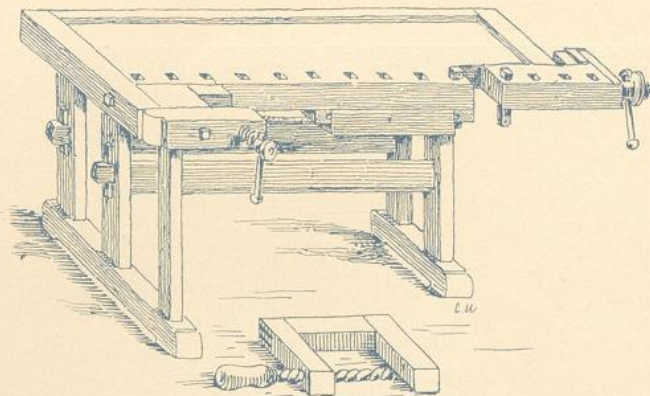
Fig. 56. Hobelbank und Schraubzwinge.
