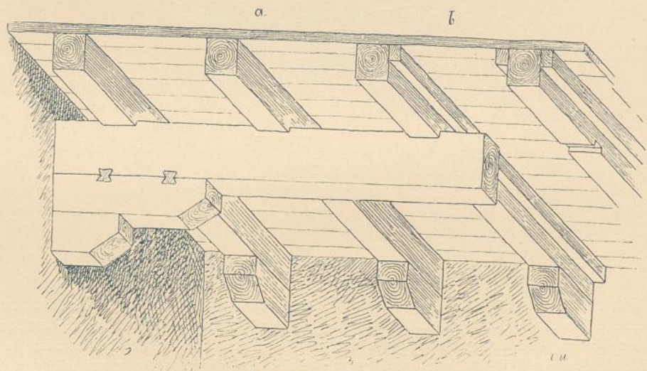
Fig. 79. Balkendecke mit Träger.
