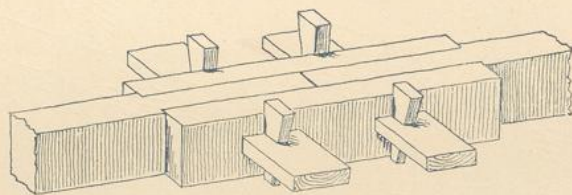
Fig. 70. Verlängerung auf Stein- unterlage.
