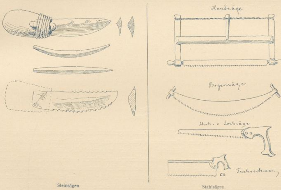
Fig. 53. Sägen.
