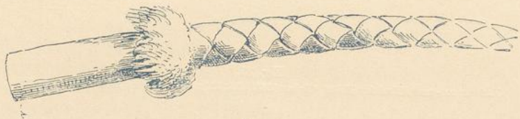
Fig. 40. Peitschenstiele.
