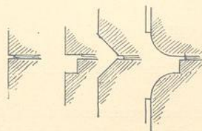
Fig. 173. Fuge.
