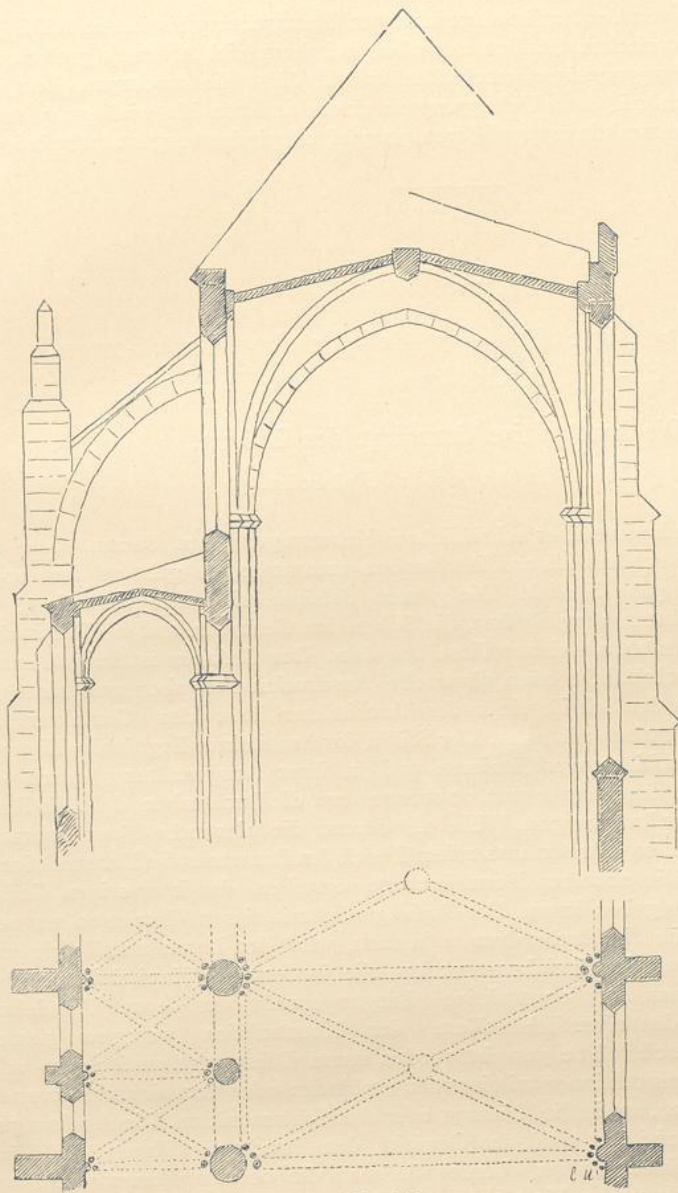
Fig. 146. Gotische Baukonstruktion.
