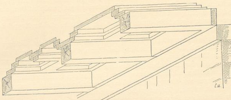
Fig. 138. Holzbalkendecke.
