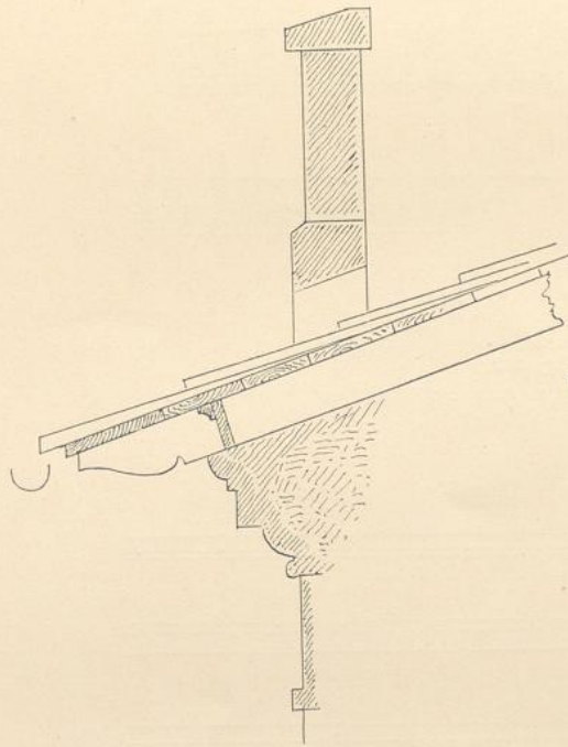
Fig. 214. Hauptgesimse mit Dach und Attika.
