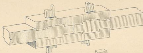
Fig. 71. Freitragende Längsver- bindungen.
