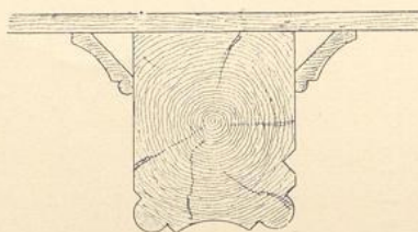
Fig. 265. Mittelalterliche Balkendecke.
