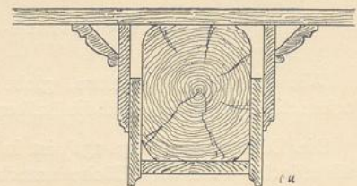
Fig. 264. Mit Brett umkleideter Balken.
