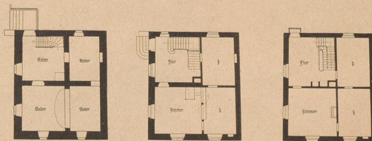
Ensisheim. Milchgasse 21, Haus Häbig. Von 1735. Grundrisse Keller, Erdgeschoss, Obergeschoss.
