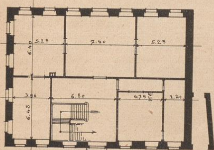
Grundriß. Erdgeschoß.
