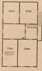
Grundriß Obergeschoß.
