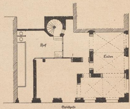
Strassburg. Ecke Spiegelgasse und Münsterplatz (1528) Erd- und Obergeschoss-Grundriss.
