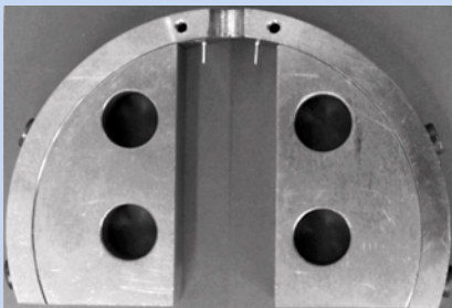
Sonderprobe zur bruchmechanischen Charakterisierung von Rohrwerkstoffen
