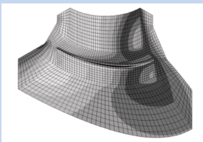
Finite Elemente Modell zur Bestimmung der Spannungen und Verformungen in einer Mischerschaukel
