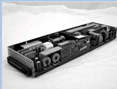
Stromversorgungseinheit für ein Serversystem informationstechnischer Anlagen der Telekommunikations- und Datenzentren.
