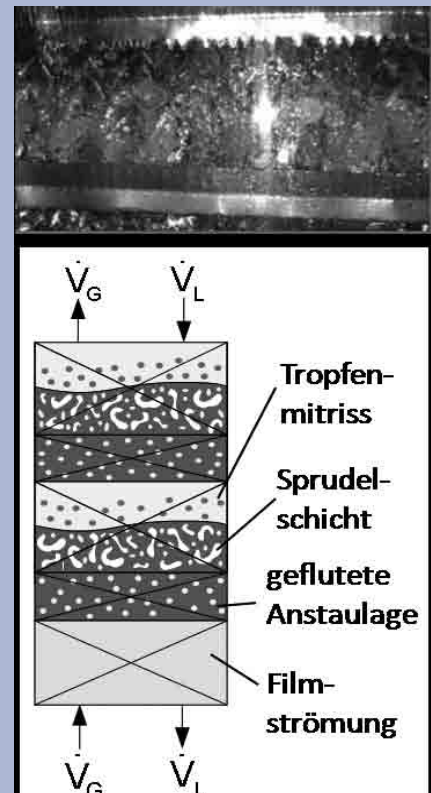
Eine Weiterentwicklung von strukturierten Packungen für den Einsatz in Rektifikationskolonnen stellen Anstaulagen dar. Oben: Aufnahme der Strömung in einer gefluteten Packung. Unten: schematische Darstellung einer Rektifikationskolonne mit Anstaulagen.
