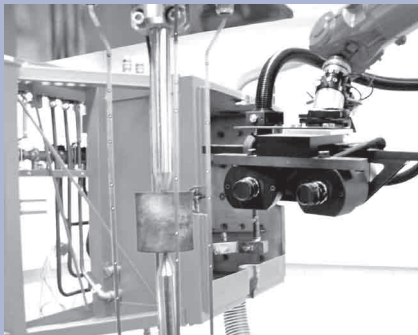
Automatische 3D-Vermessung einer deformierten Struktur
